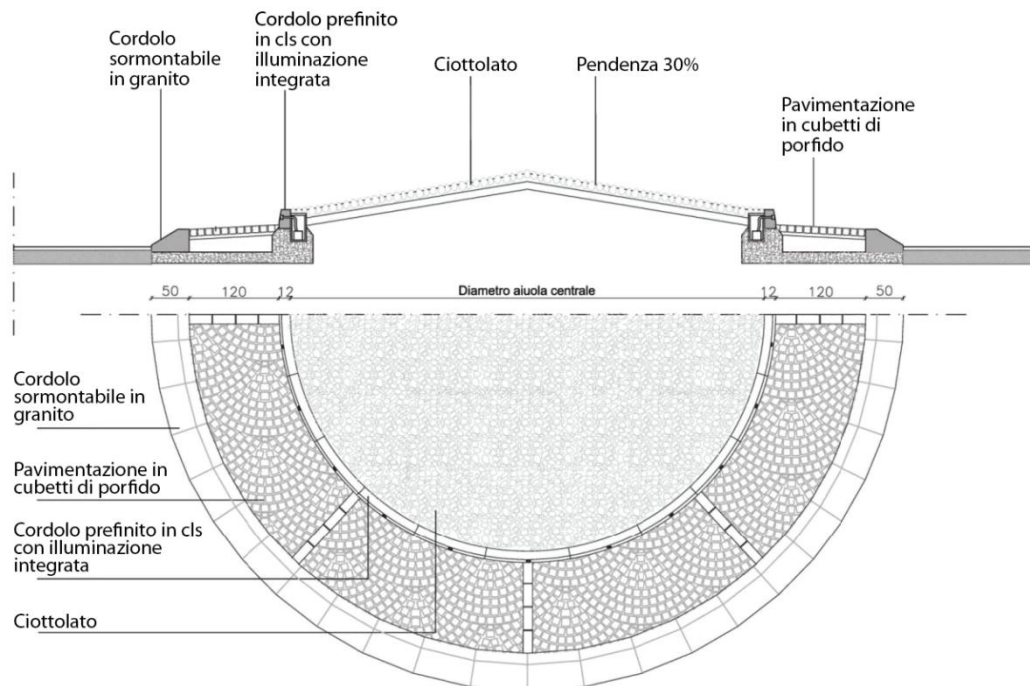
Mini rotatoria con isola circolare centrale in parte transitabile (18ml < diam < 25 ml)
