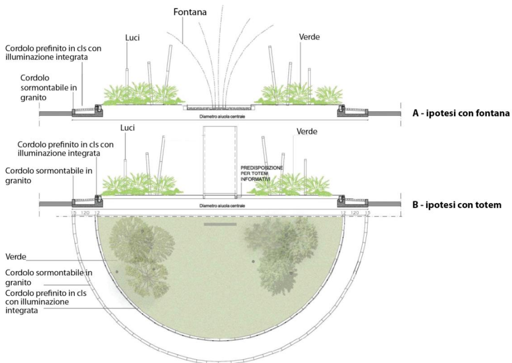
Rotatoria convenzionale ( 40\text{ ml} < \text{diam} < 50\text{ ml} ). Ipotesi di allestimento aiuola centrale: A con verde, illuminazione e fontana; B – con verde, illuminazione e totem manifestazioni.
