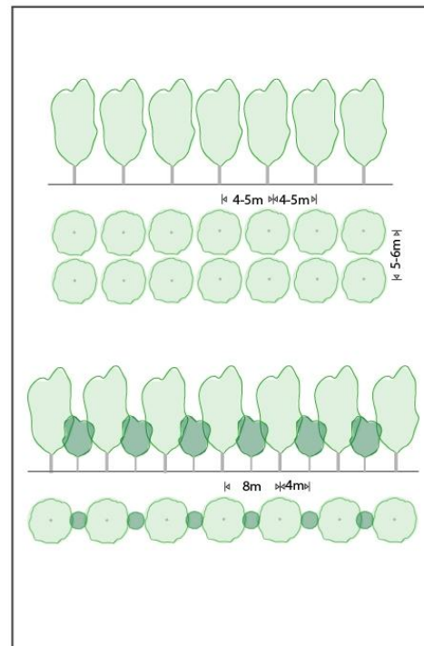
Filari alberati - impianti composti con specie di seconda e terza grandezza
