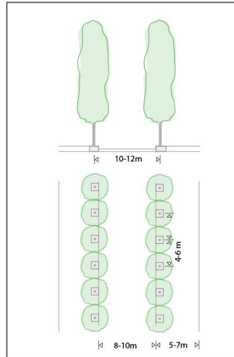
Filari alberati su viali stretti con specie di prima grandezza a portamento fastigiato
