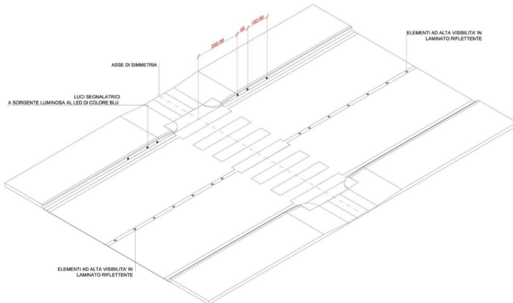
Attraversamento pedonale a raso. Strada a due corsie con doppio senso di marcia
